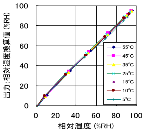
相対湿度-出力特性
