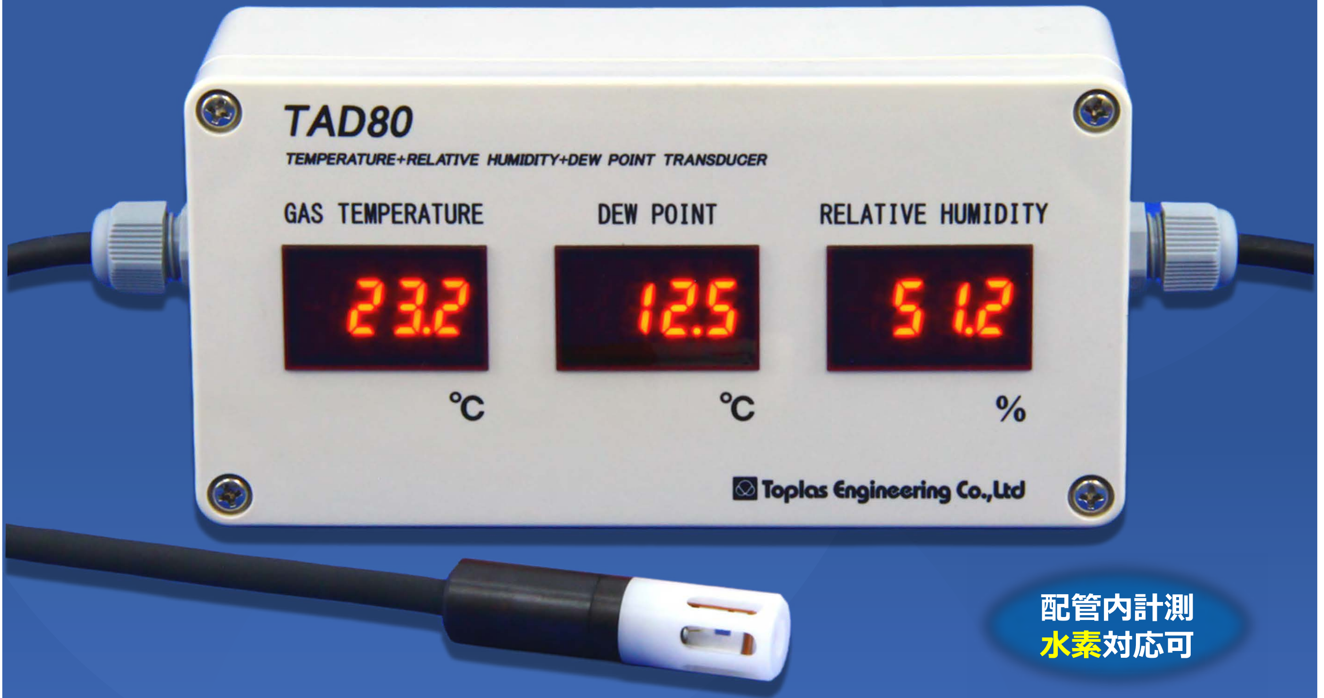
TAD80 (センサ部形状:標準型、LED表示器:有り)
